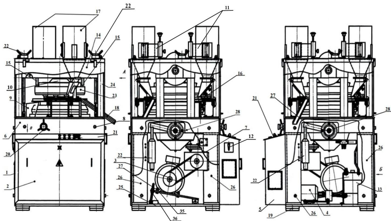
Рисунок 1 Загальний вид
